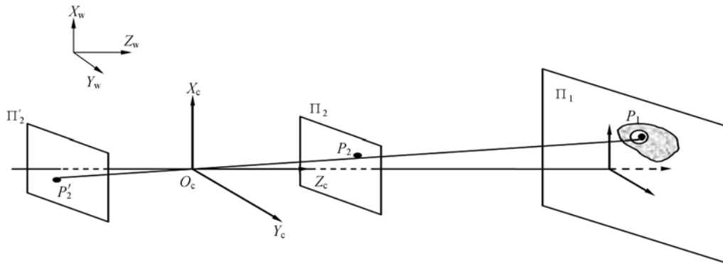
图 1 小孔成像原理图 Fig. 1 Pinhole camera model
