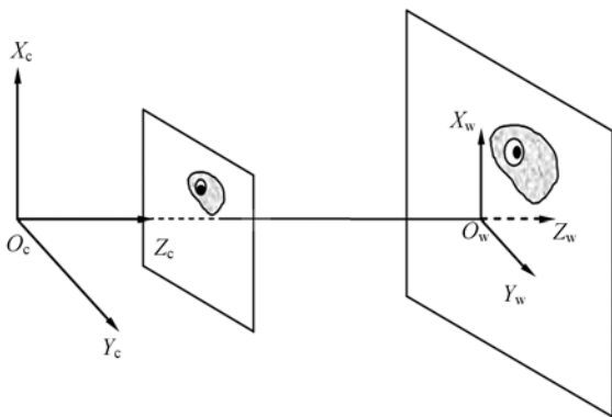
图 2 垂直于光轴中心线平面内目标的测量 Fig. 2 Distance measurement of object in plane
