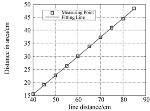
图 5 目标平面内距离测量误差分析
